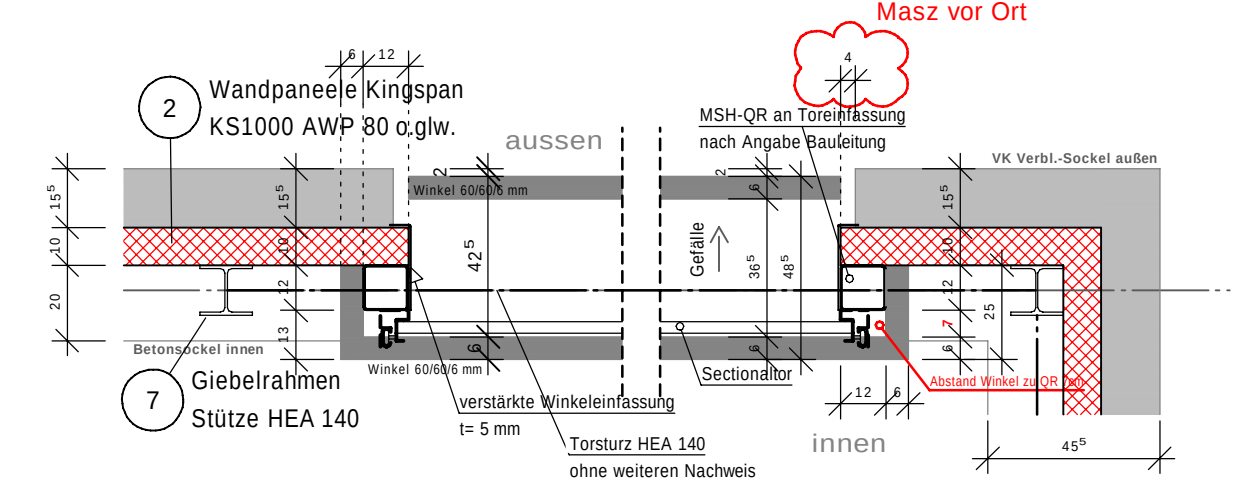
DETAIL 6-6 HALLE: Torabschluss M: 1:20
