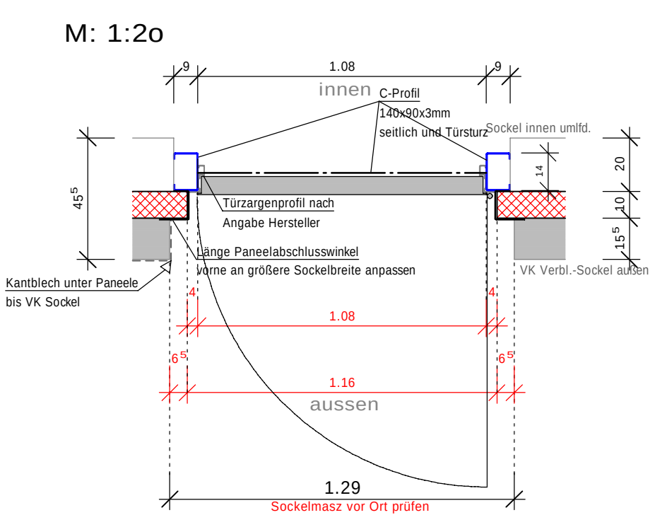
DETAIL 8-8 Halle: Türdetail
